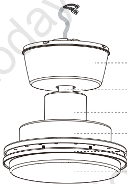
3. Canopy
